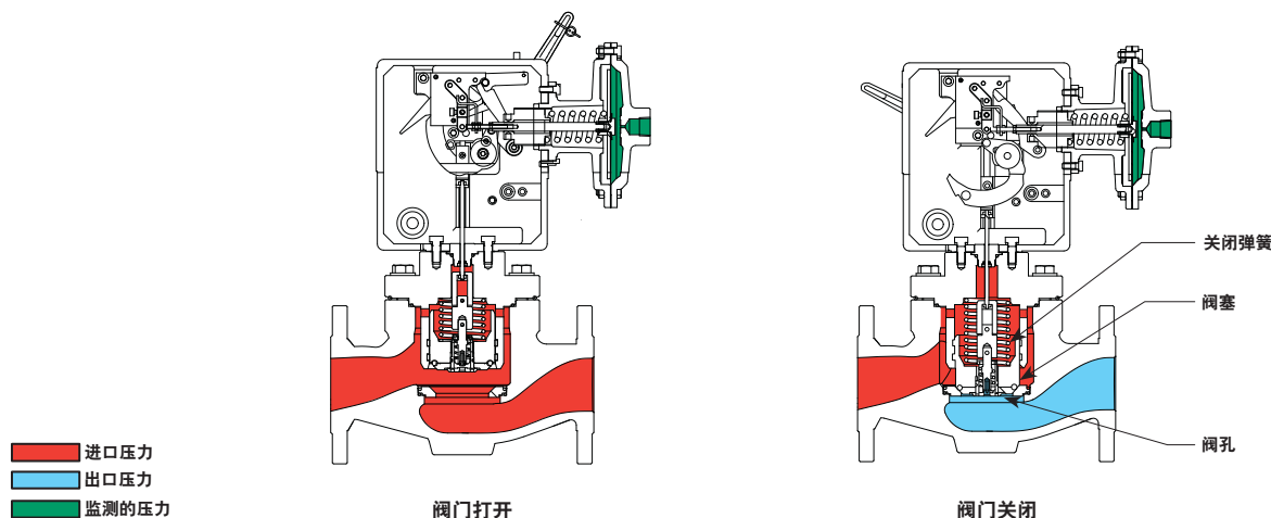
图3. JEQ型运行示意图
