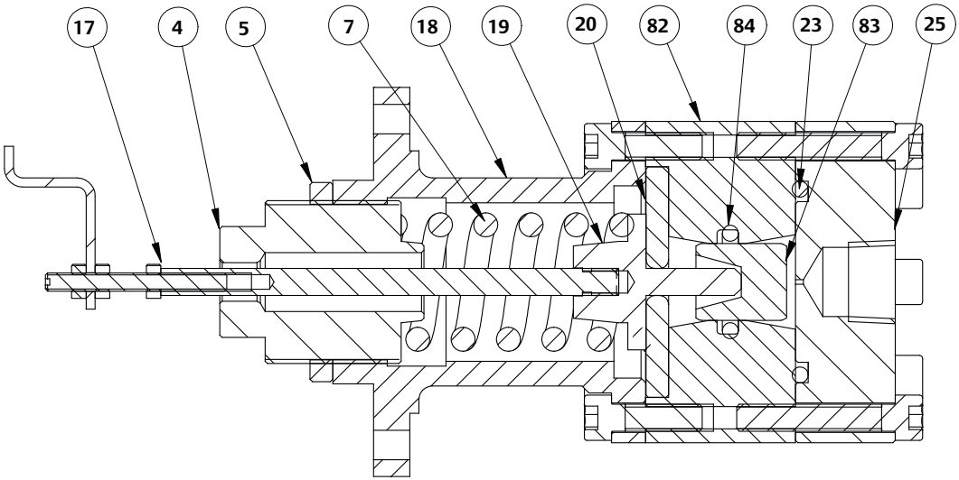
图19. D型测压感应设备 (BMS)
