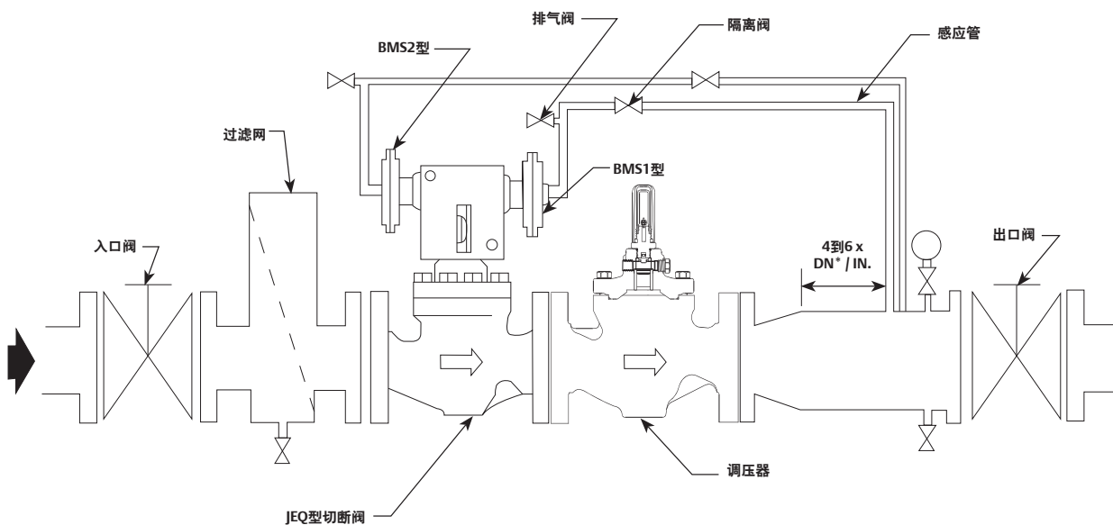
图6. 使用两个测压感应设备（BMS1型和BMS2型）进行超压和失压关闭
