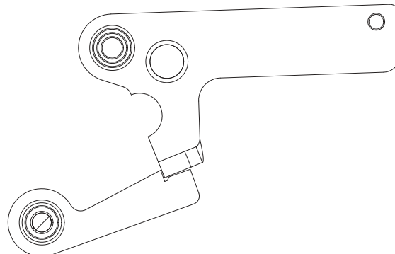
图14. BMS2型结构
