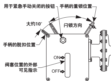
图8. JEQ型重锁位置和方向（前视图）
