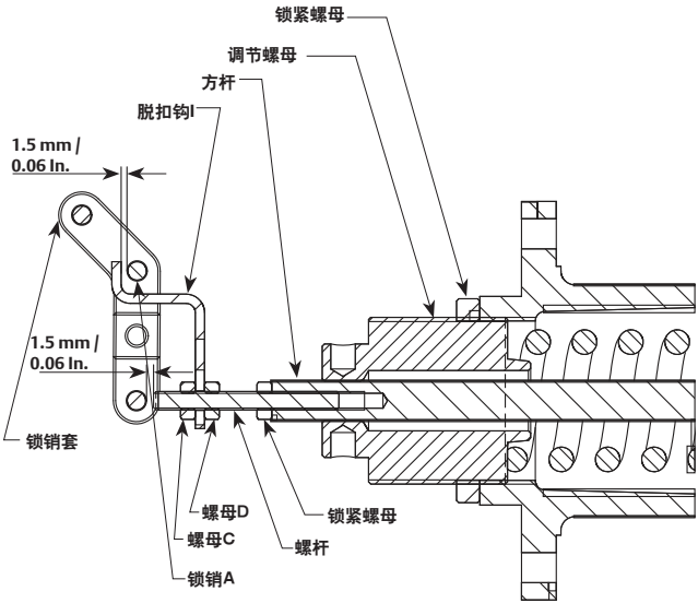
图10. BMS1型结构
