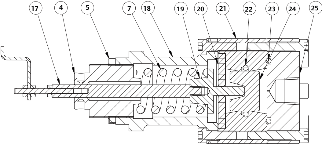
图18. C型测压感应设备 (BMS)
