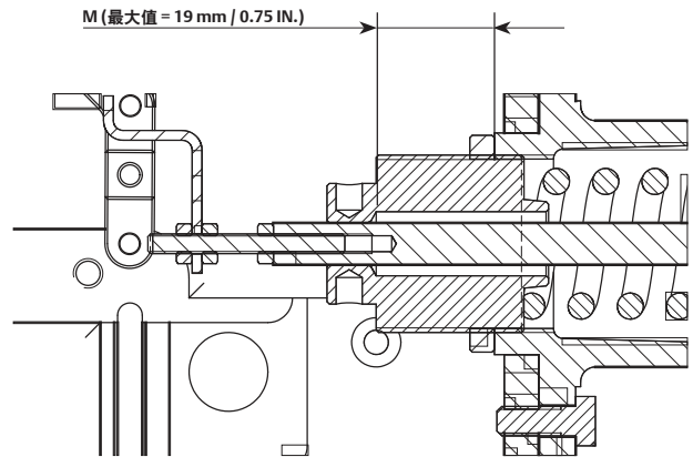
图15. 调节螺母从弹簧箱中拧出的最大长度M
