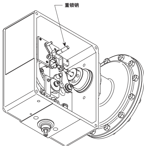
图11. 位于检测机构中的重锁销
