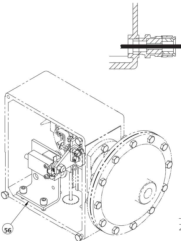
图22. 远程警报（只用于“关闭位置”，带电缆接头）
