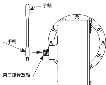
图7. JEQ型重锁位置和方向（侧视图）
