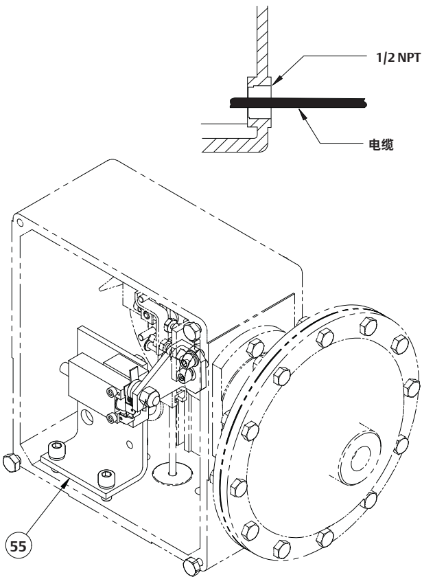
图21. 远程警报（只用于“关闭位置”，无电缆接头）
