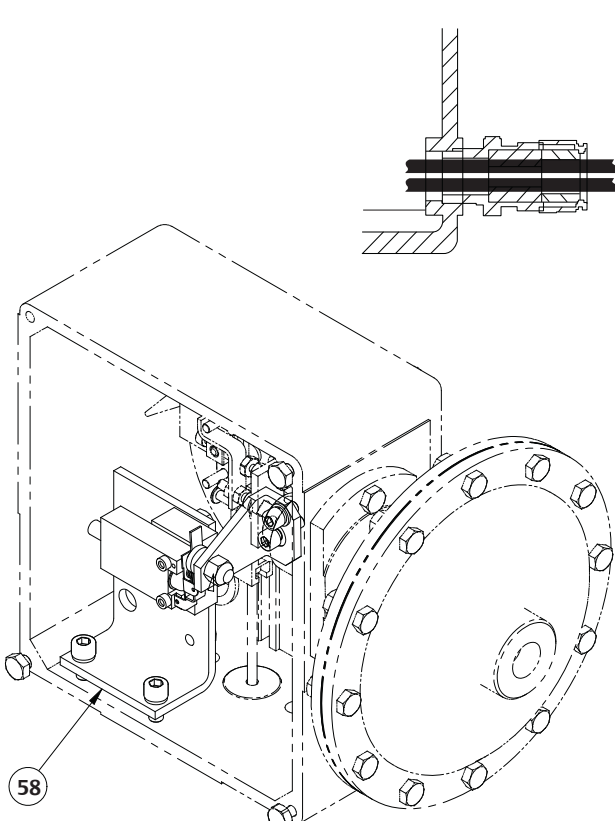
图24. 远程警报（用于“打开位置”和“关闭位置”，带电缆接头）
