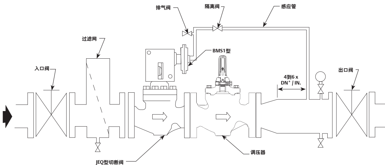
图5. 只使用一个测压感应设备（BMS1型）进行超压和失压关闭
