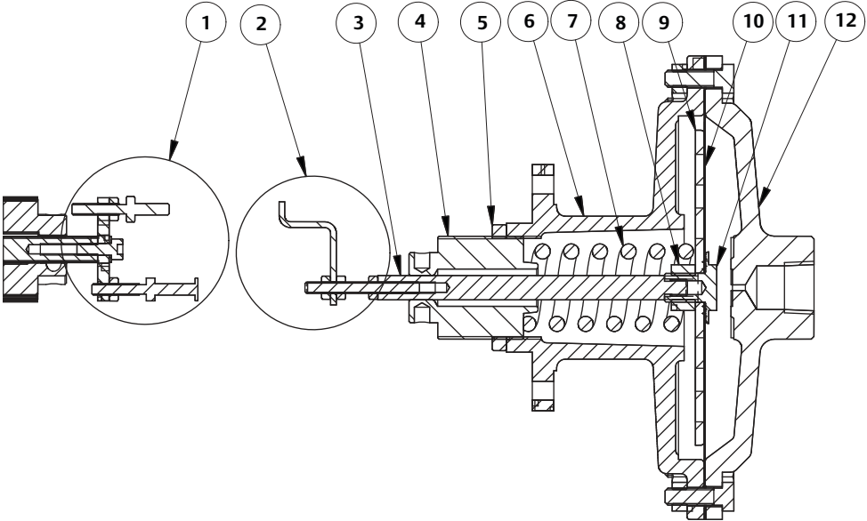
图17. B型测压感应设备 (BMS)
