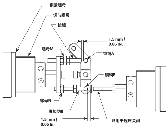
图14. BMS2型结构
