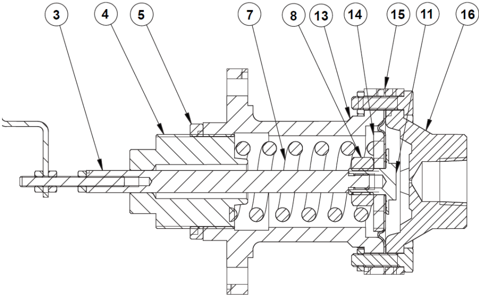
图18. C型测压感应设备 (BMS)
