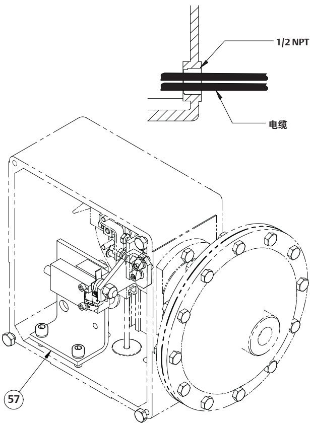
图23. 远程警报（用于“打开位置”和“关闭位置”，无电缆接头）
